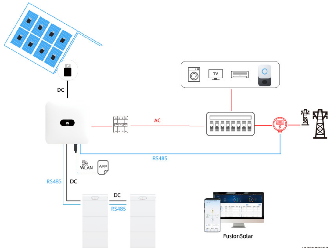
Abbildung 2-7 Netzgekoppeltes Szenario
